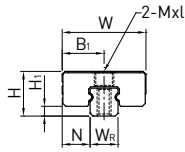
MGN2
