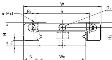
MGW14
