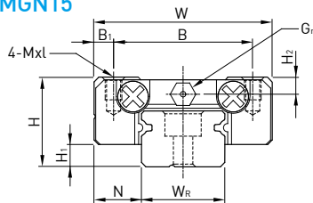
MGN15
