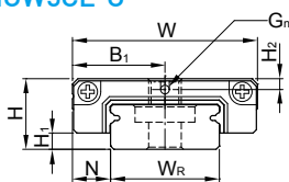
MGW5CL-0
